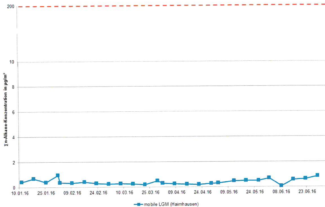
Abbildung 24. Verlauf der Summe der gemessenen n-Alkan-Konzentration der mobilen LGM für den Messzeitraum 11.01.16 - 04.07.16 [Wochenmittelwerte, hilfswise herangezogener Beurteilungswert für Innenräume von 200 µg/m 3 rot gestrichelt markiert].
