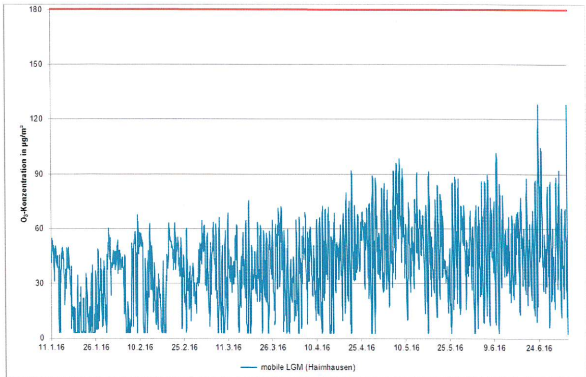
Abbildung 22. Verlauf der gemessenen O_3 -Konzentration der mobilen LGM für den Messzeitraum 11.01.16 – 04.07.16 [Stundenmittelwerte, O_3 -Stundeninformationsschwelle 180 \mu\text{g}/\text{m}^3 rot markiert].
