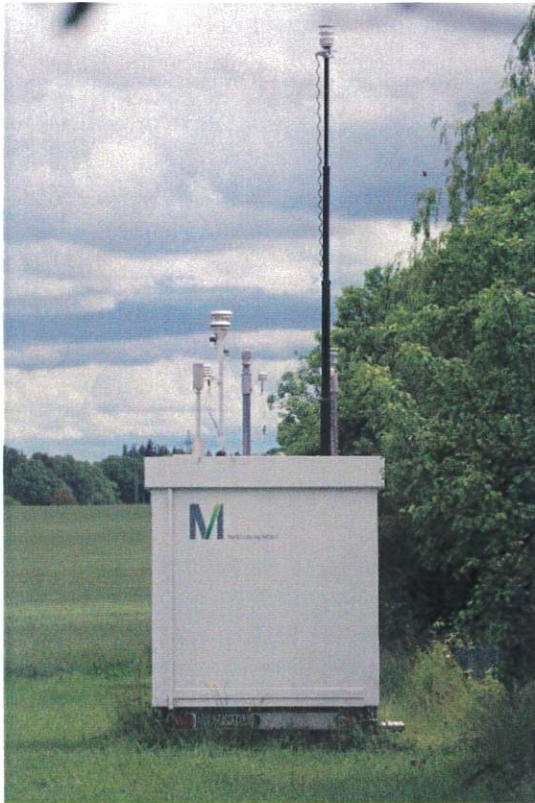
Abbildung 10. Außenansicht der mobilen Luftgütemesstation am Standort „östlich Mischgebiet“ in Haimhausen.
