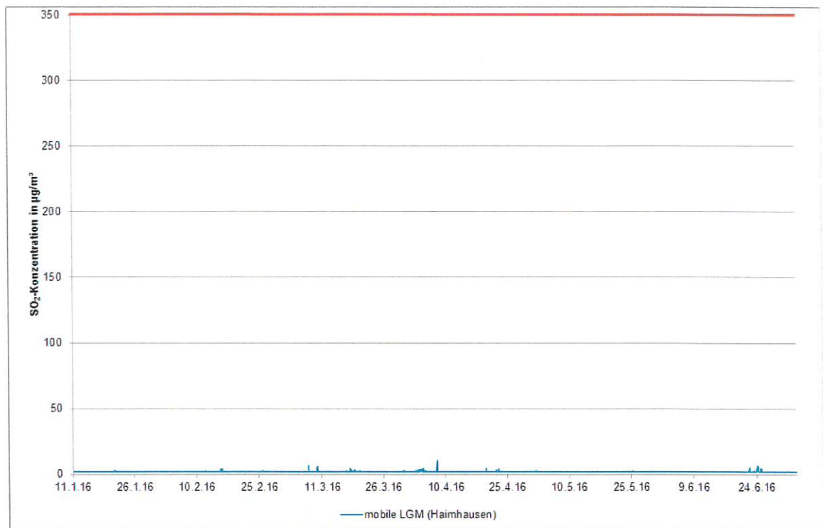
Abbildung 21. Verlauf der gemessenen \text{SO}_2 -Konzentration der mobilen LGM für den Messzeitraum 11.01.16 - 04.07.16 [Stundenmittelwerte, \text{SO}_2 -Stundengrenzwert 350 \mu\text{g}/\text{m}^3 rot markiert].
