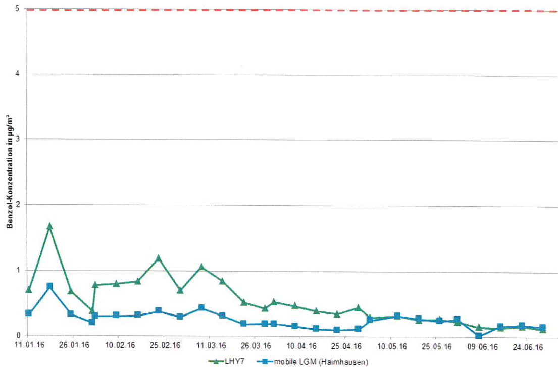
Abbildung 34: Verlauf der Benzol-Konzentration der mobilen LGM und der Hauptmessstation LHY7 für den Messzeitraum 11.01.16 - 04.07.16 [Wochenmittelwerte, Immissionsgrenzwert 5 \mu\text{g}/\text{m}^3 rot gestrichelt markiert].
