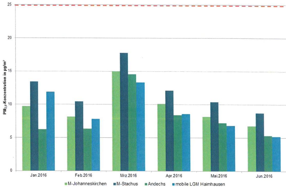
Abbildung 38: Vergleich der PM 2,5 -Monatsmittelwerte LÜB – mobile LGM Haimhausen (Monatsmittelwerte, PM 2,5 -Jahresgrenzwert 25 µg/m 3 rot gestrichelt markiert).
