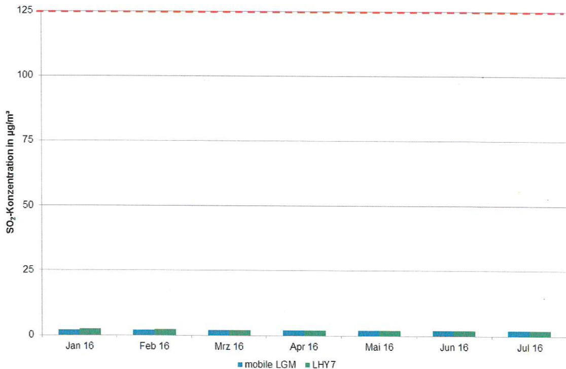
Abbildung 32: Verlauf der SO 2 -Konzentration der mobilen LGM und der Hauptmessstation LHY7 für den Messzeitraum 11.01.16 - 04.07.16 [Monatsmittelwerte, Grenzwert für das Tagesmittel 125 µg/m 3 rot gestrichelt markiert].
