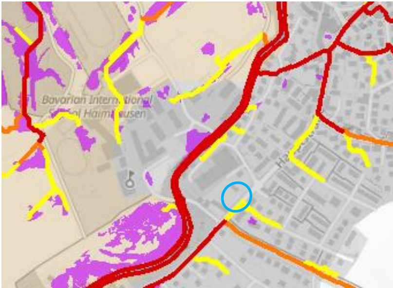
Abb. 8 Hinweiskarte Oberflächenabfluss und Sturzflut – ohne Maßstab Quelle: LfU
