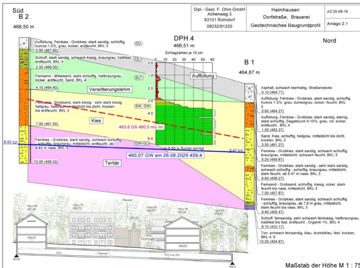
Abb. 16 Baugrundprofil mit Gründungssohle und Grundwasserstand – ohne Maßstab Quelle: Ohin GmbH
